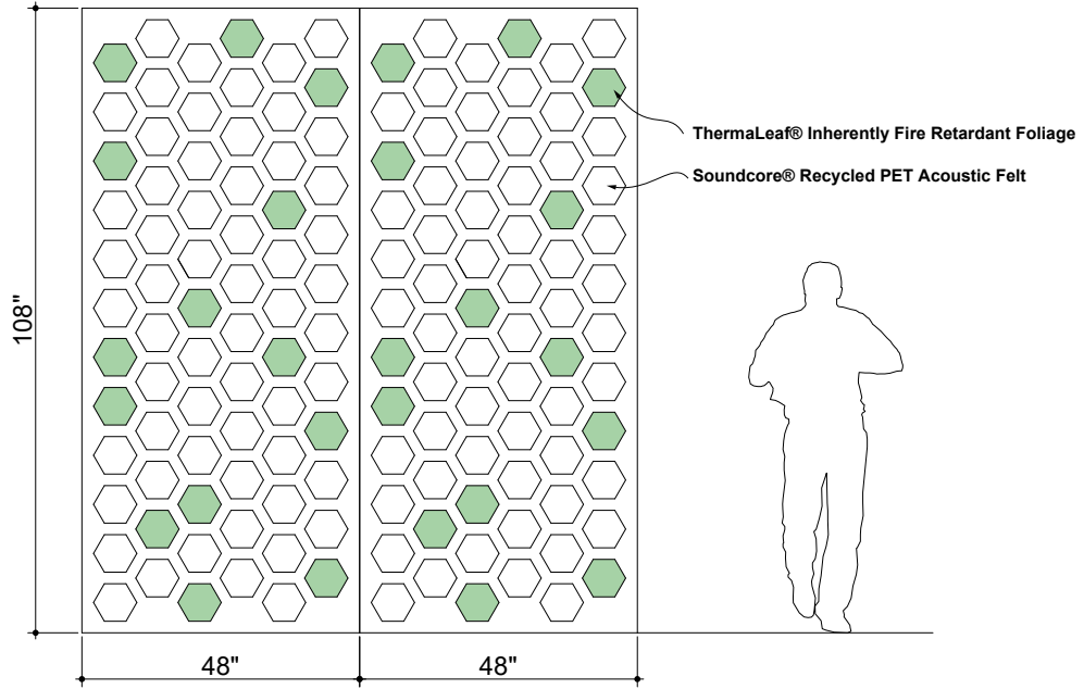
① ELEVATION 1
