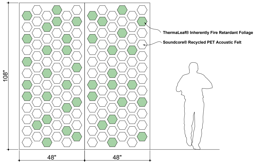
② ELEVATION 2
